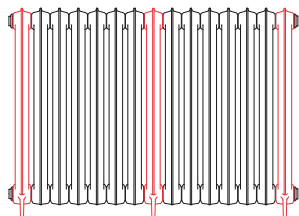
920 x 1262 15 sekcji (3+12)
