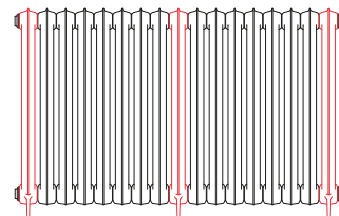
920 x 1426 17 sekcji (3+14)
